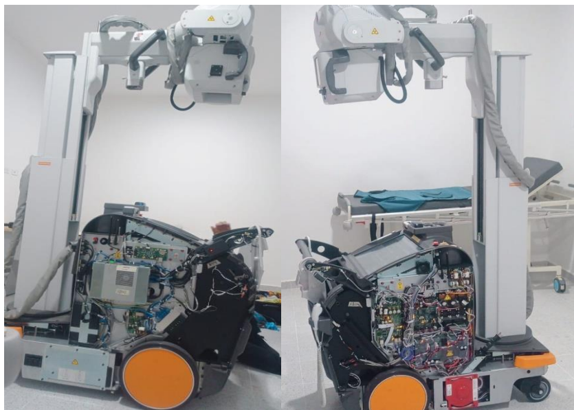
Figura [11]. Equipo de rayos x portátil.
